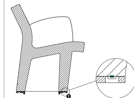
Sección | Section
