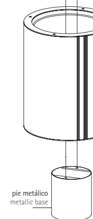
tornillos M-10 screws M-10
