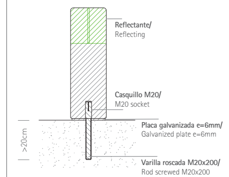
Sección A'A' | Section A'A'
