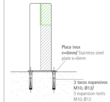
Sección AA | Section AA
