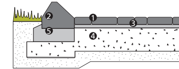
Sección AA | Section AA
