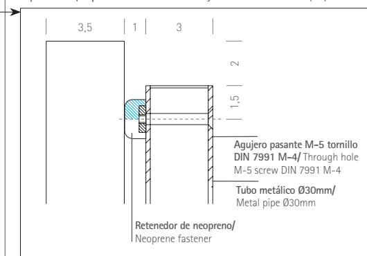
Detalle sección | Detail section
